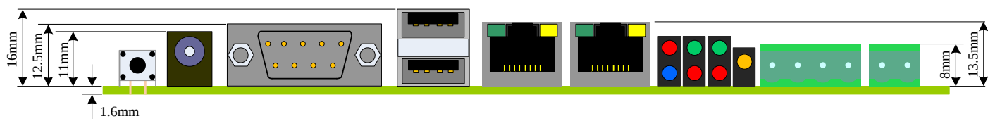
图 2: ESMARC EVB 端口布局图及尺寸 (单位: mm)
