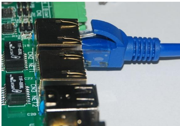
将开发主机和 ESM6800 接入以太网
