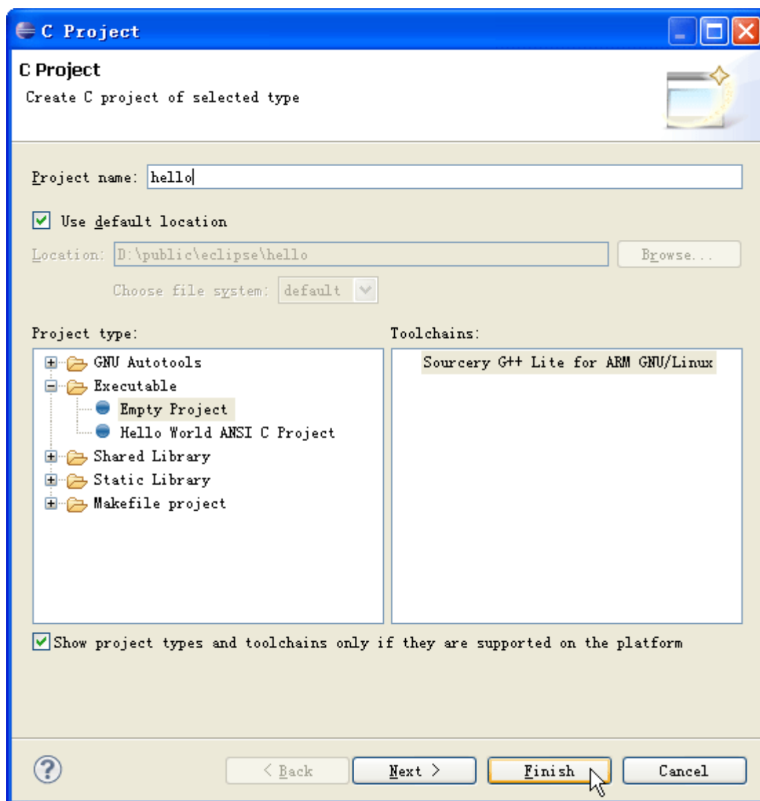
选择 Toolchains
