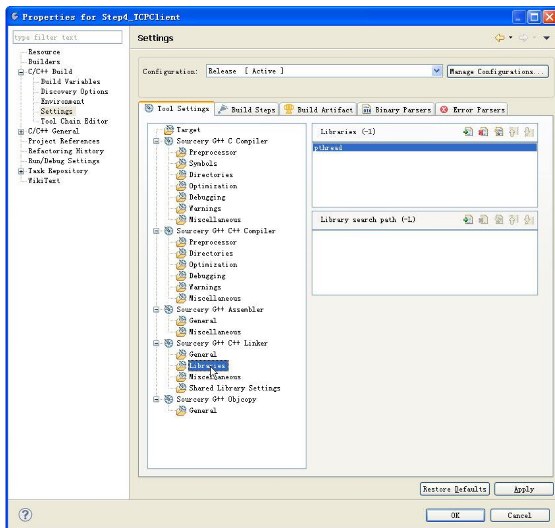
设置库连接
