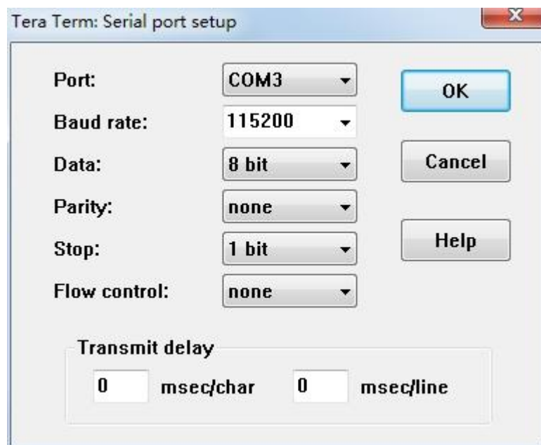
COM3 参数配置
