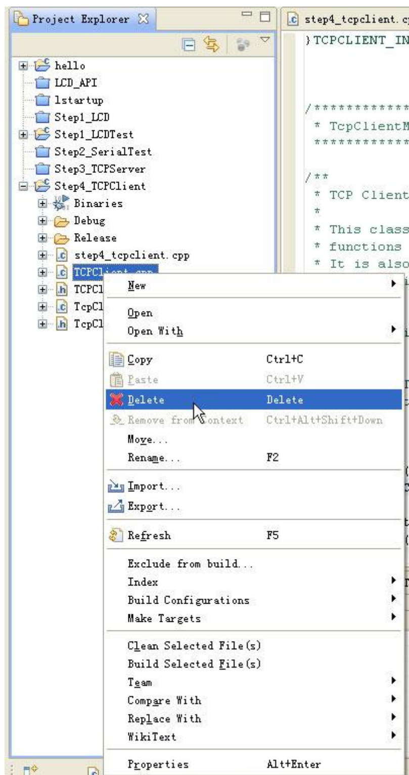
删除源文件
