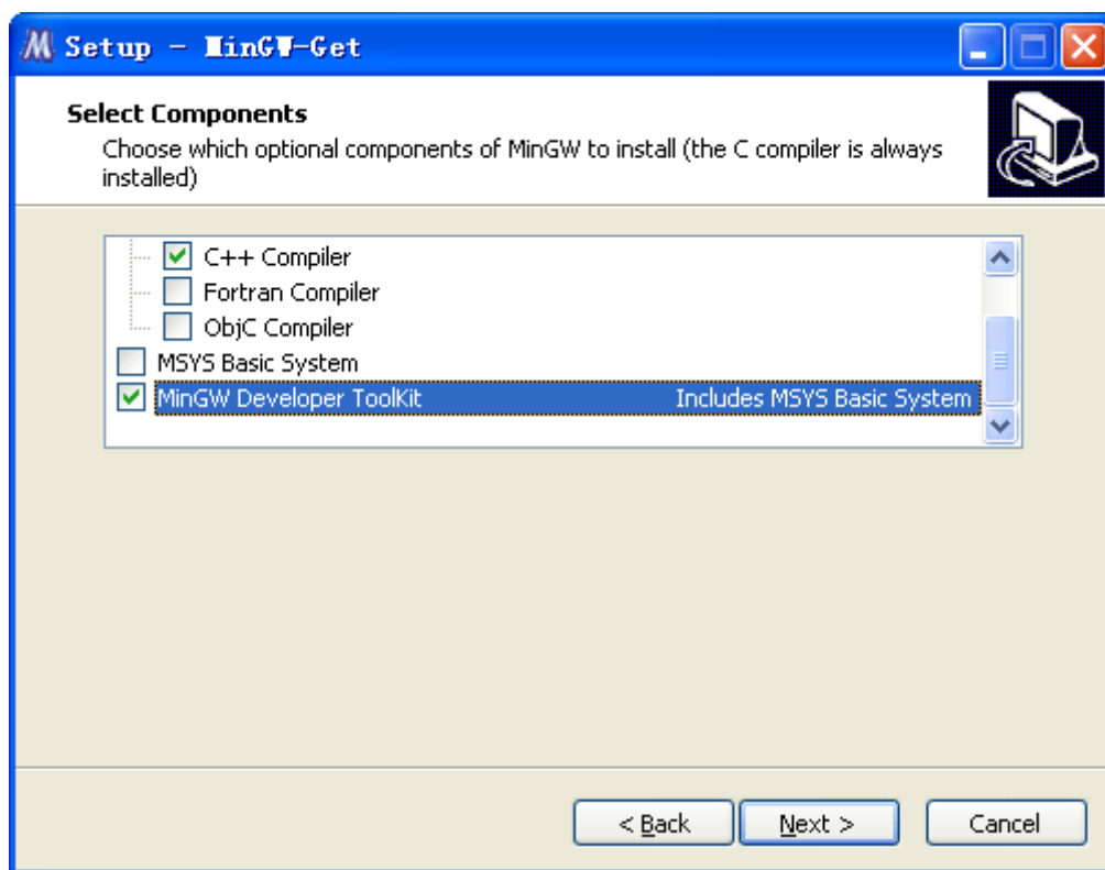
安装 MinGW
