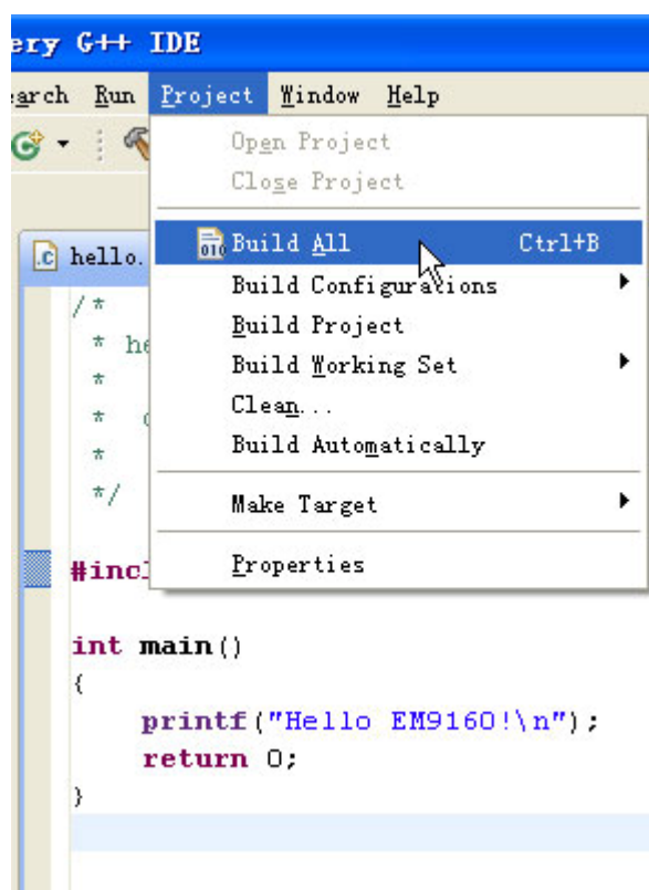
编译源码
