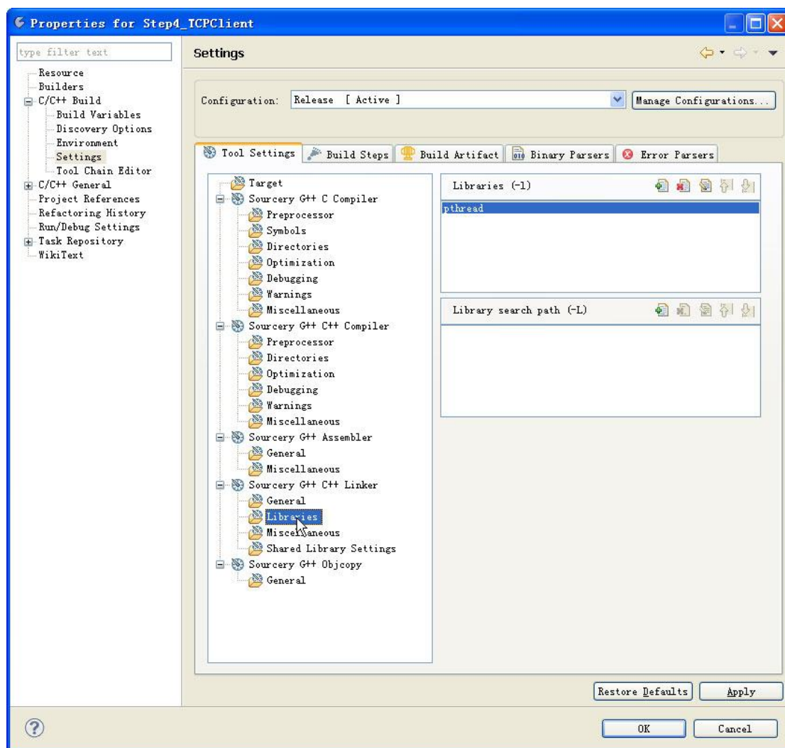
链接库文件
